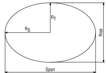
Fig. 4 - Ellipse
